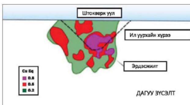
Штокверк уул дахь концепцийн судалгааны ил уурхай ба блок малталтын зураг
